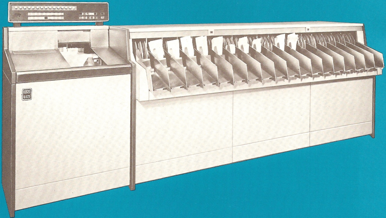
671-101 MICR Sorter/Reader
